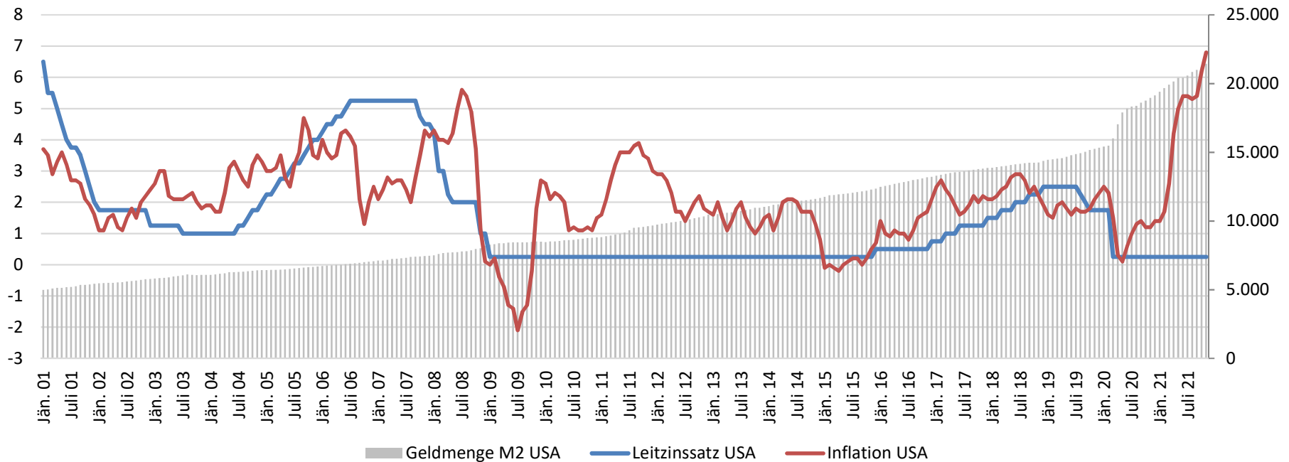
Geldmenge M2, FED-Leitzinssatz und Gesamt-Inflation in den USA
